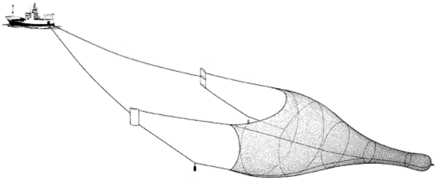
Midwater seine
